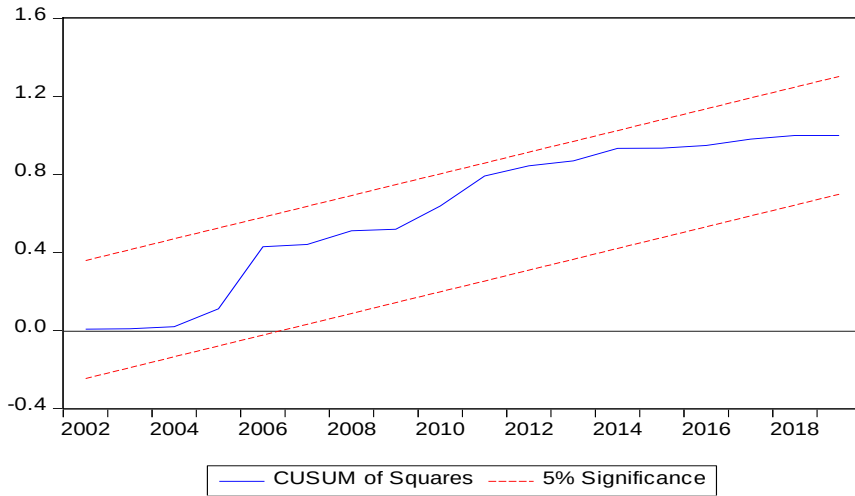
Şekil 6 – CUSUMSQ Grafiği
