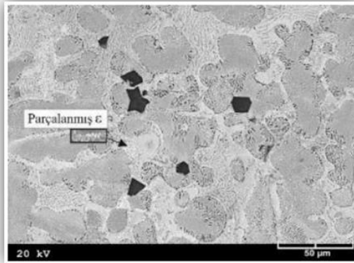
Şekil 7. Zn-15Al-3Cu-1Si alaşımının T5 ısı işlemi sonrası mikroyapısı (Savaşkan ve Hekimoğlu, 2011: 430).
