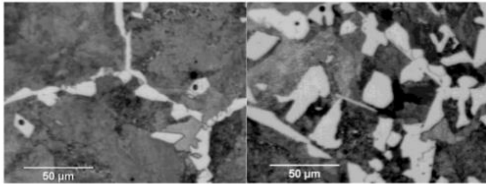
Şekil 5. 1200°C'de ısıtılmış F alaşımını (sol) ve E alaşımını (sağ) (Cryderman vd.; 2015: 768).
