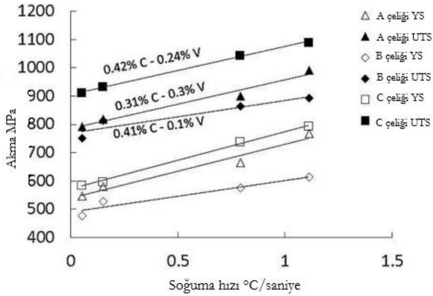
Şekil 8. Farklı soğutma hızlarının çekme (UTS) ve akma (YS) dayanımına etkisi (Cryderman vd.; 2015: 768).
