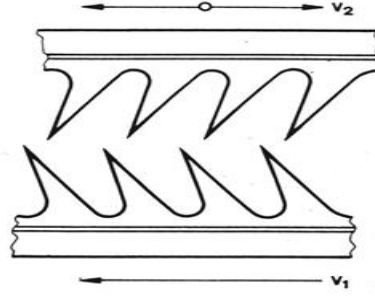
Şekil 11. Garnitür tellerinin sıyırma pozisyonundaki konumları (Klein, 2011: 26)
