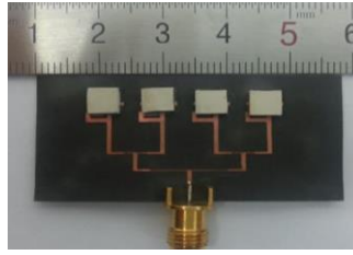
Şekil 2 - Önerilen küp şeklinde dielektrik rezonatöre sahip yama anten tasarımı (Nor vd., 2016:58-59).
