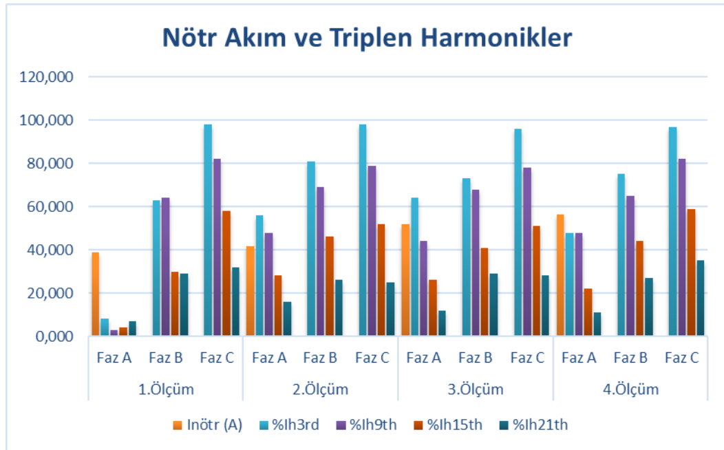
Şekil 4. Tüm ölçümler için üç fazda nötr akım, %THD 13 , %THD 19 , %THD 115 ve %THD 121 değişimi
