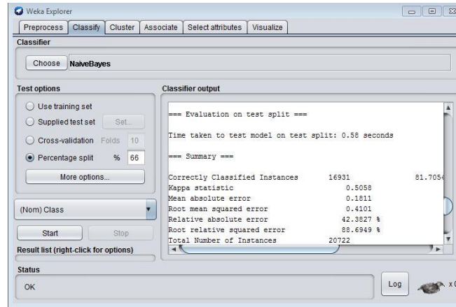
Şekil 1: Weka Sonuç Ekranı
