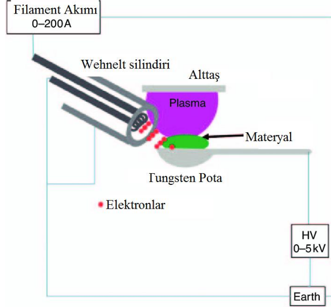
Şekil 5. TVA sistemi şematigi
