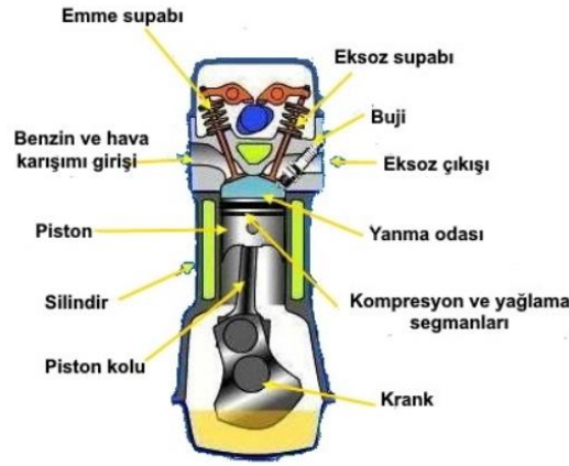
Şekil 1. Biyel kolunun motor içerisindeki konumu (Çetinerler, E., Erişim Tarihi (22.04.2022), ( http://www.havaciyiz.com/Kutuphane03-Piston.htm ))
