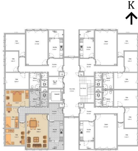
Şekil 10. Yapsat Yöntemiyle Yapılan Plan Örneği (URL-7)
