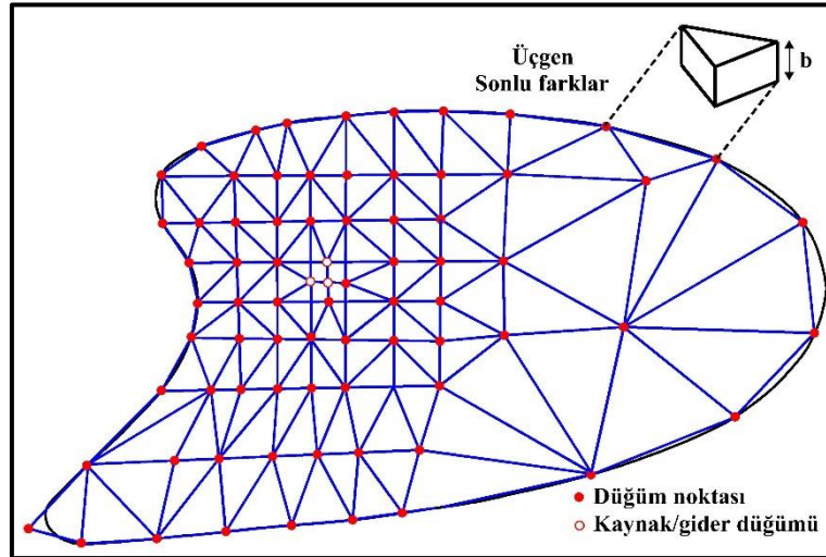
Şekil 4. b akifer kalınlığındaki akifer çalışması için sonlu elamanlar düzeni (Thomas, 1992).
