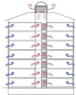
Şekil 7. Merkezde Düzenlenen Merdiven ve Hava Akımı İlişkisinin Şematik Gösterimi, 2022 (Yazarlar tarafından üretilmiştir)
