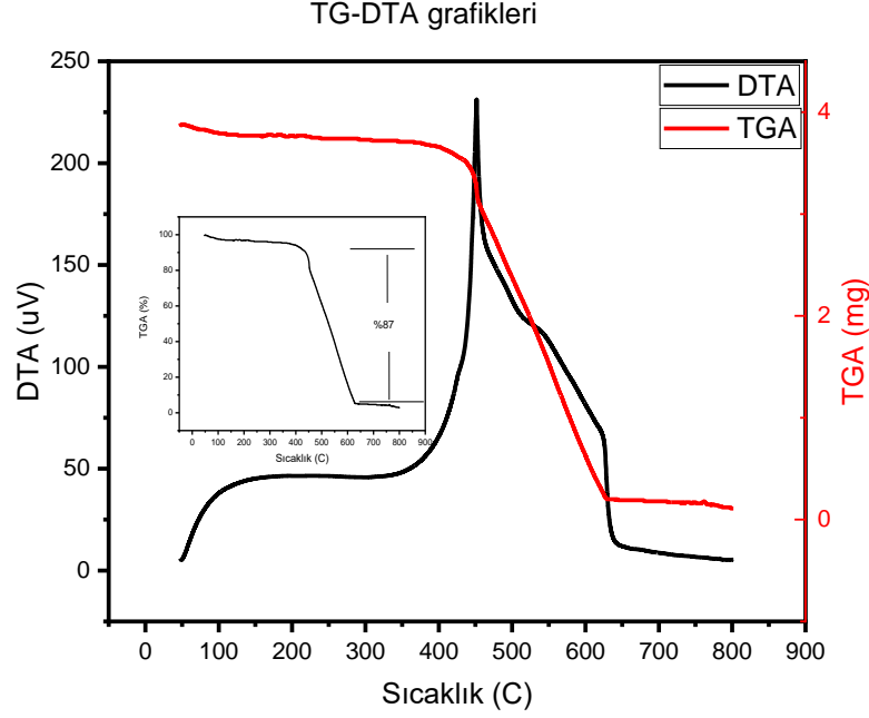
Şekil 3. DTA-TG eğrisi.
