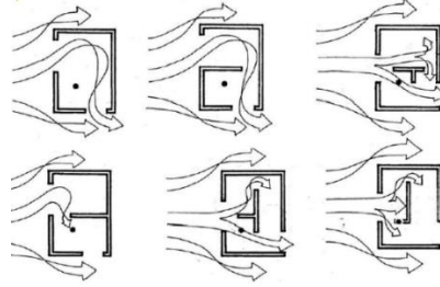
Şekil 6. Hava Akım Bölgesinde Yer Alan Bölme Duvarına Göre Mekanın Havalandırma Şeması (Zorer, 2016)
