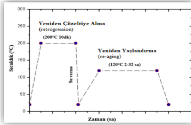
Şekil 9. RRA ısl çevrim diyagramı (Altuntaş ve Bostan, 2021: 5).
