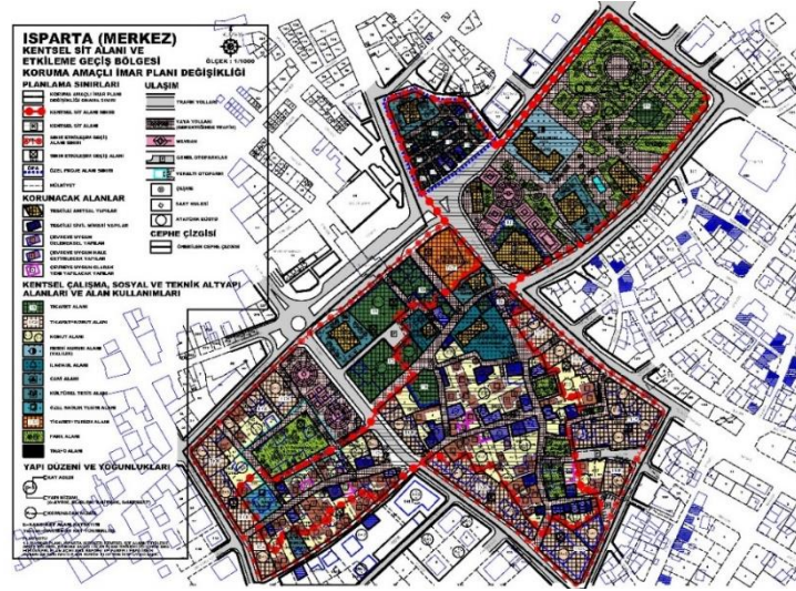
Şekil 14. Tarihi Kent Merkezi Koruma Amaçlı İmar Planı
