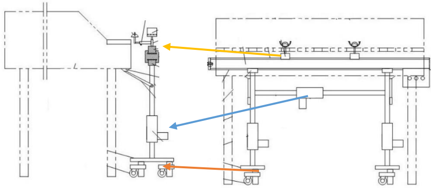
Resim 1. Piyano Çalışması için El Tıpi Düzeltme Cihazı'nın çizimleri (Hualing ve Erjun, 2019).
