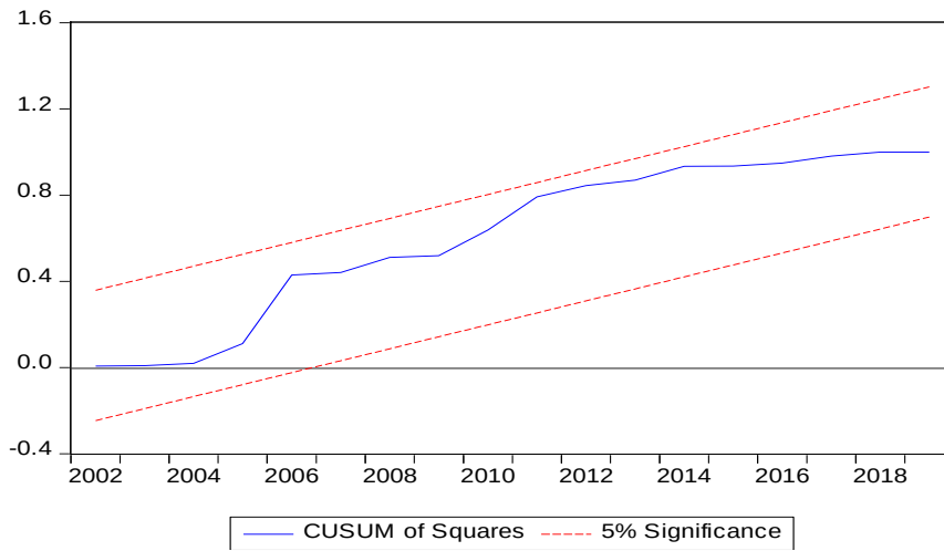
Şekil 6 – CUSUMSQ Grafiği
