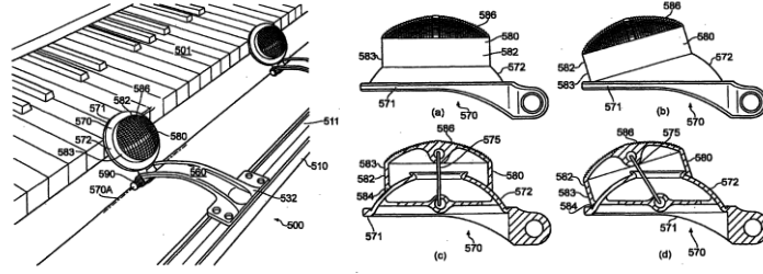
Resim 3. Klavye Alıştırma Aparatı'nın farklı eklentileri (Russell, 2008).
