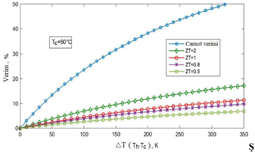
ekil 3. Bi_2Te_3 için farklı zT değerlerinde tipik TE veriminin sıcaklık farkı ile değişimi (Champier, 2017)
