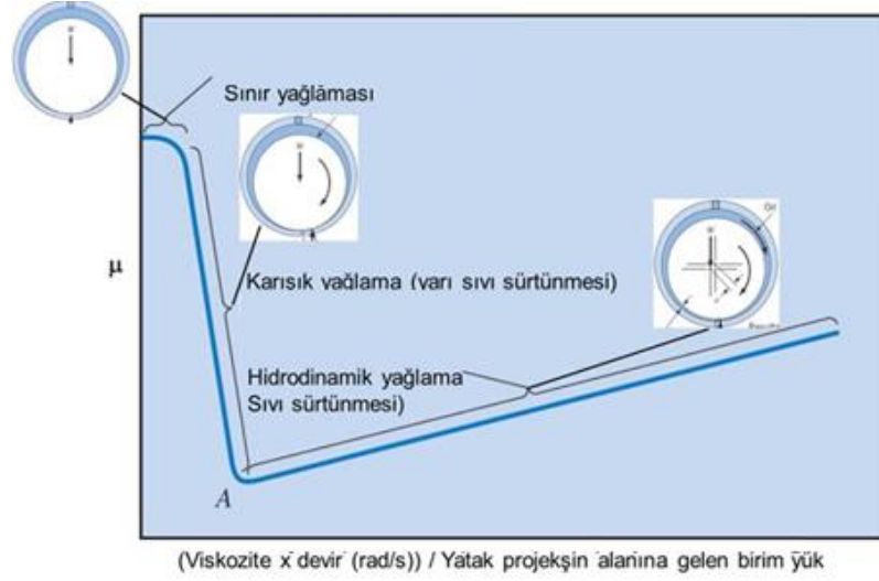
Şekil 3.4. Stribeck eğrisi ( Anonim,2010)
