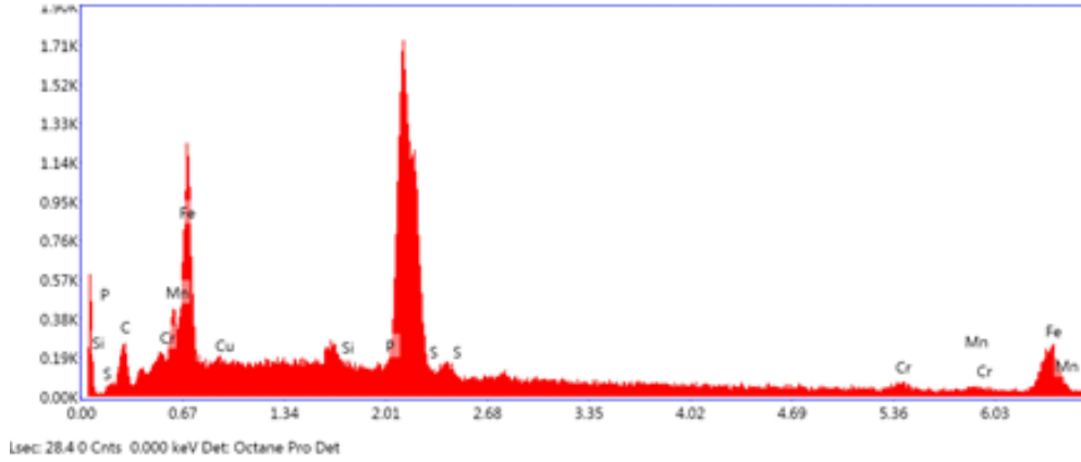
Şekil 3.2. 41Cr4 Çeliğinin ham numunesinden (41-H1) alınan EDS analiz pikini.
