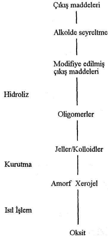
Şekil 2 Sol-Jel Yönteminin Akış Şeması
