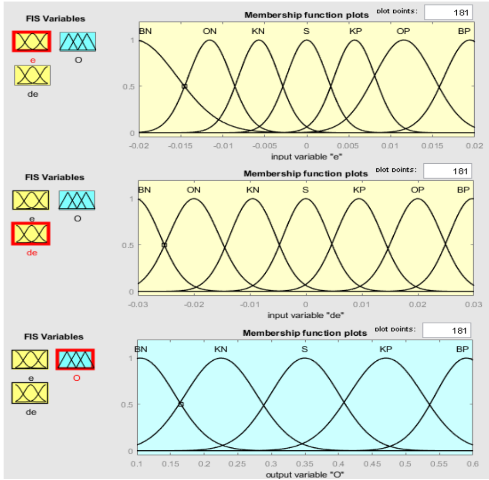
Şekil 11. Bulanık-PI giriş-çıkış üyelik fonksiyonları.
