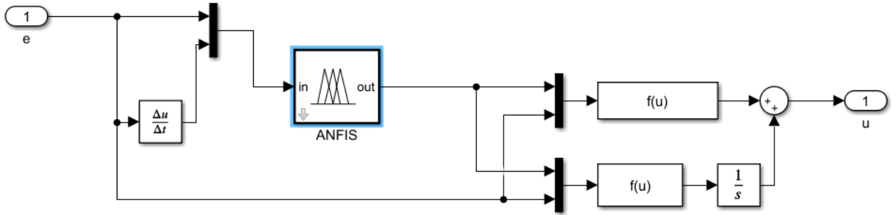
Şekil 15. ANFIS_PI kontrolör MATLAB modeli.
