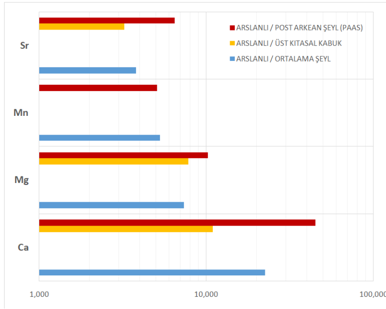
Şekil 6. Aslanlı sahası bitümlü kayaçlarında karbonat minerali yapıcı elementlerin Üst Kıtasal Kabuğa, Post Arkean Şeyli ve Ortalama Şeyl'e göre zenginleşmeleri.
