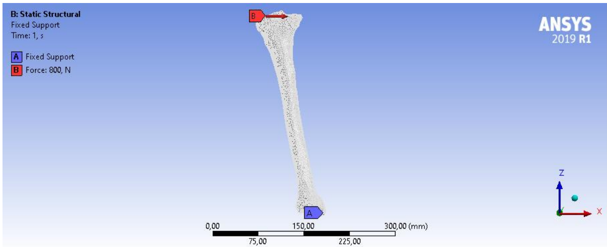
Şekil 37. Sol Tibia Kemiği X Yönündeki Sınır Şartları
