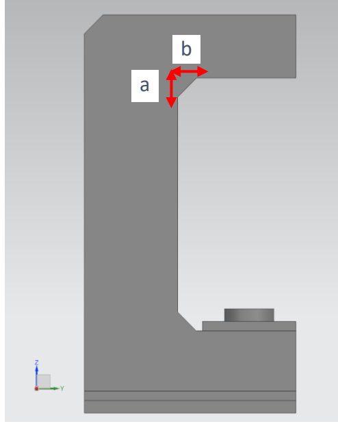
Şekil 3. C Tipi Pres Şekil Optimizasyonu için pah ölçülerinin tespiti
