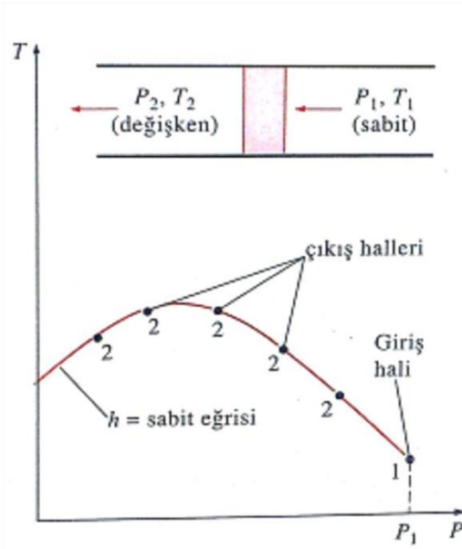
Grafik 1. P-t diyagramındaki h=sabit Eğrisinin Elde Edilmesi
