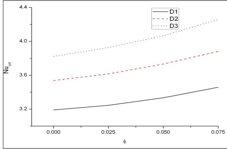
a) Gr=10^4
