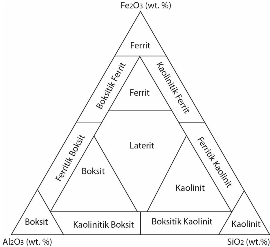
Şekil 5. SiO_2 - Al_2O_3 - Fe_2O_3 üçgen diyagramı (Aleva, 1994).
