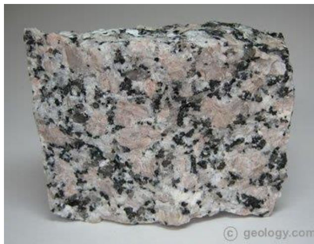
Şekil 2. Pembe ortoklas kristalleri içeren iri taneli granit örneği
