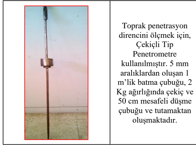
Şekil 2. Çekiçli Tip Penetrometre
