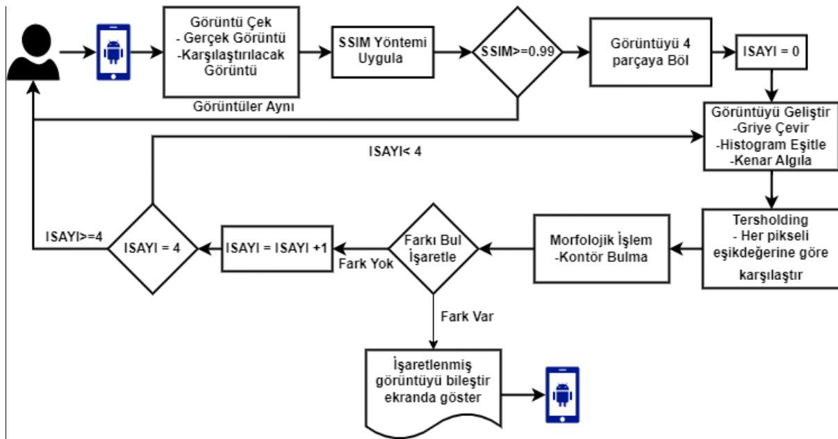
Şekil 7 Uygulama Akışı
