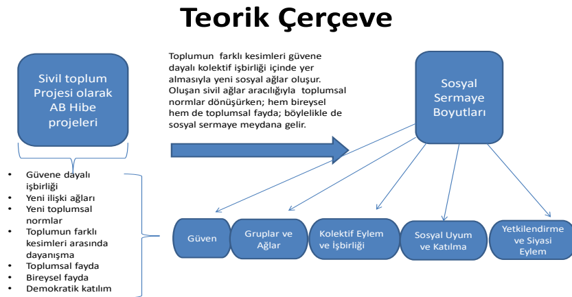
Şekil 1: Teorik Çerçeve
