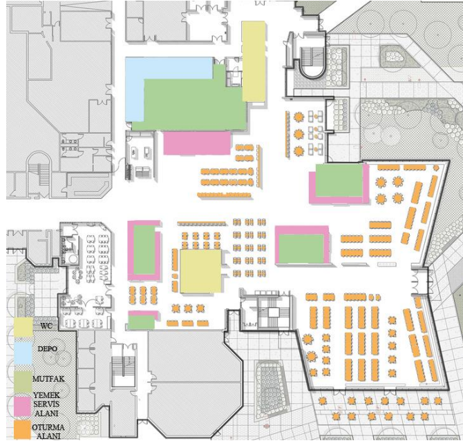
Görsel72.TomArban, Seneca College Newnham Campus Food Hall , Proje planı, 2021, Alan gösterimleri Toylor Smyth Architects'e ait olan projeden yararlanılarak 1. Yazar tarafından oluşturulmuştur, Kanada.
