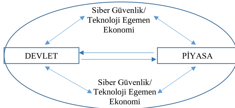
Şekil 4: Stratejinin İşleyişi
