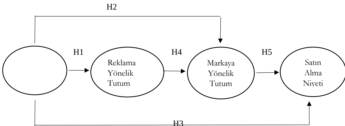
Şekil 1: Araştırma Modeli
