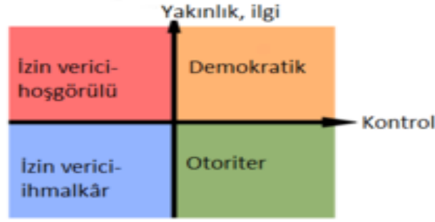
Şekil 1. Ebeveynlik Stilleri
